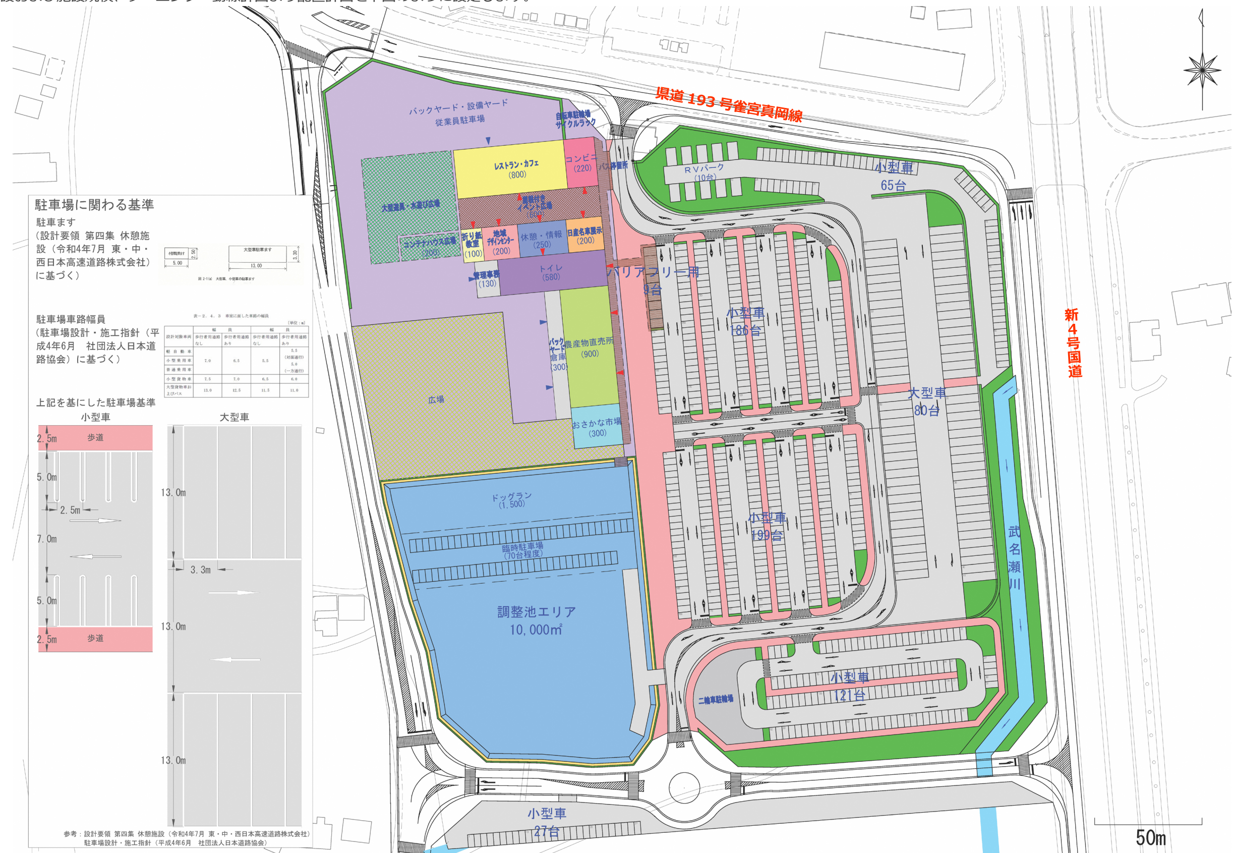
図 配置計画図
